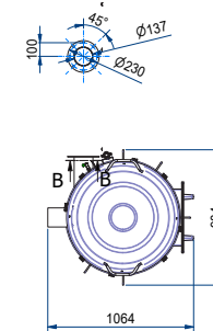
B-B ( 1:30 )
