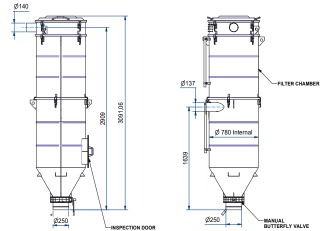
B-B ( 1:30 )
